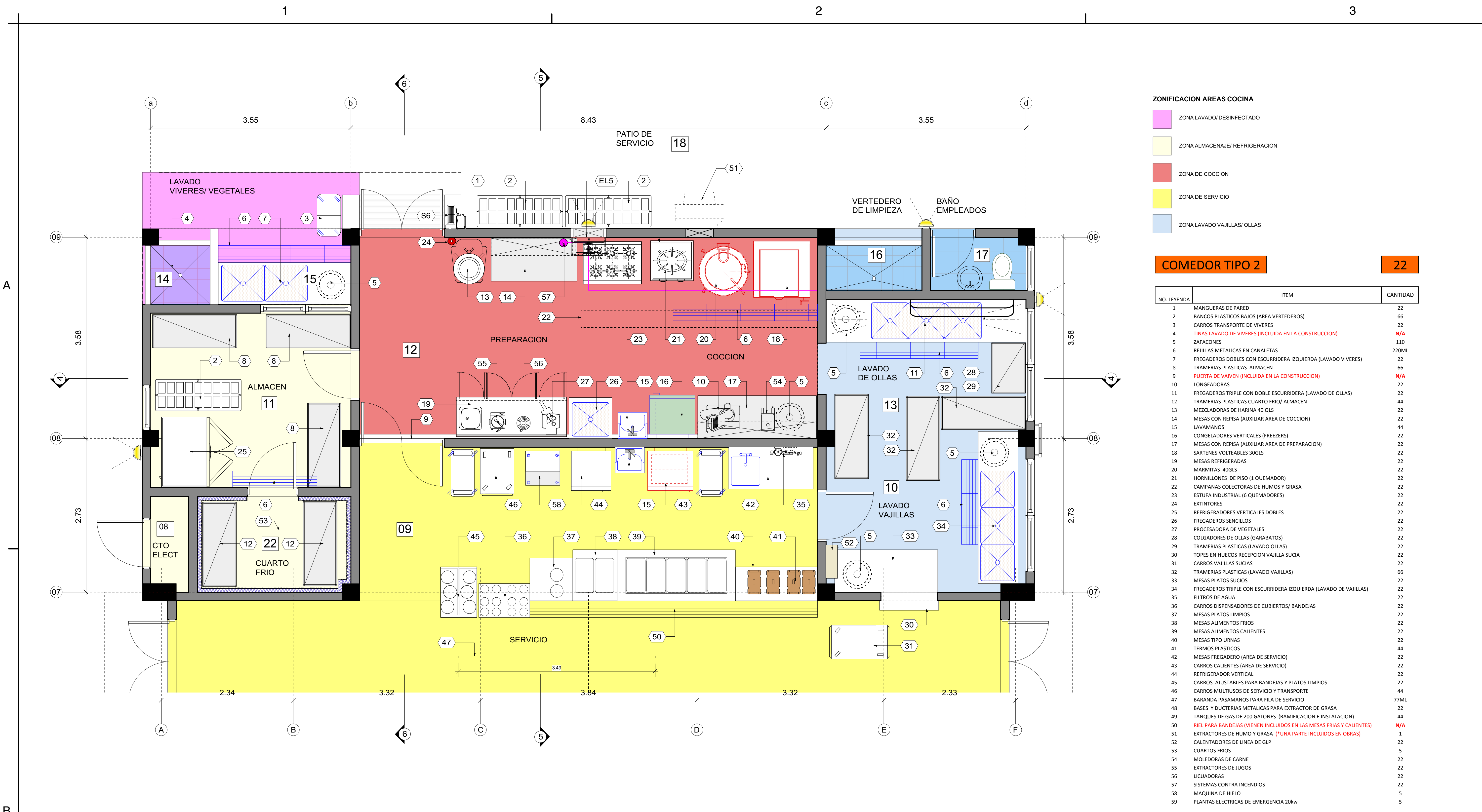
1 PLANTA DISTRIBUCION EQUIPOS COCINA TIPO 2 Scale: 1:33
