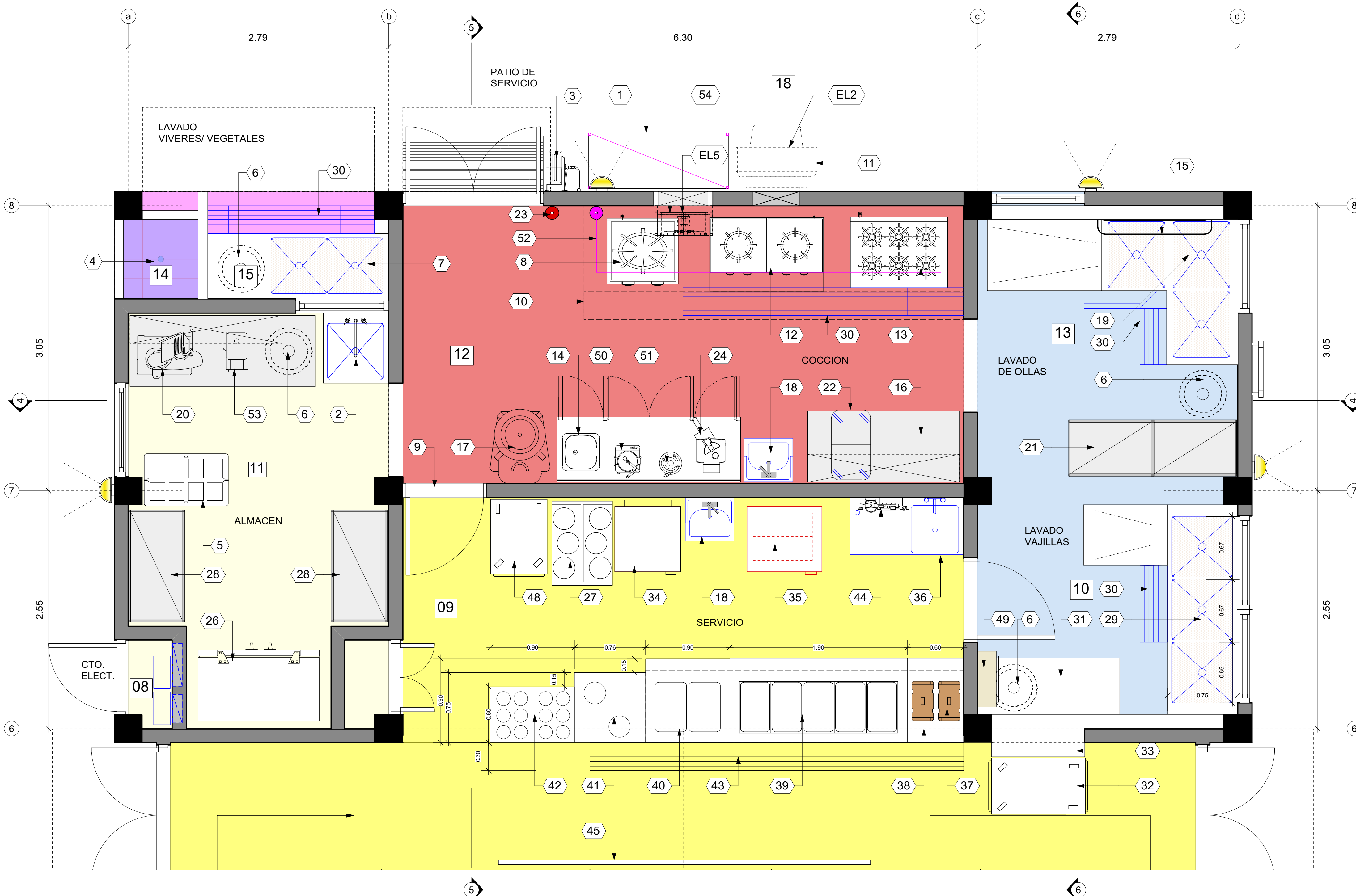
1 PLANTA COCINA COMEDOR TIPO 1 (144/TURNO) Scale: 1:25
