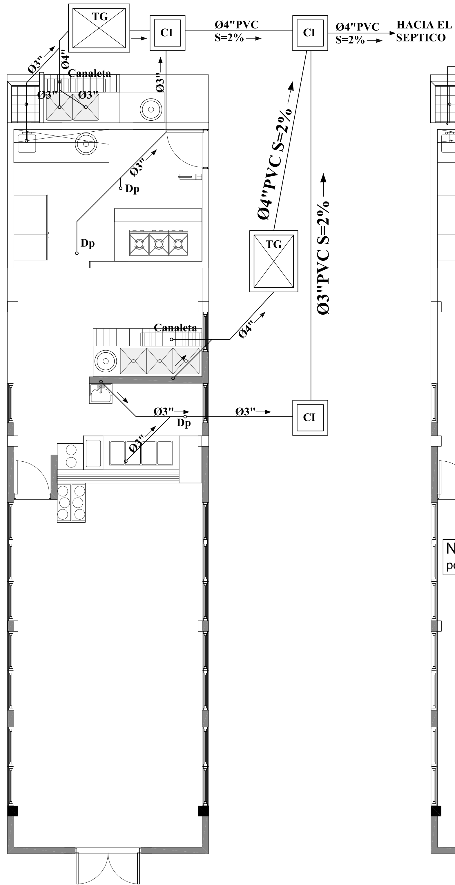
1 PLANTA SANITARIA Scale: 1:50 Aguas Residuales
