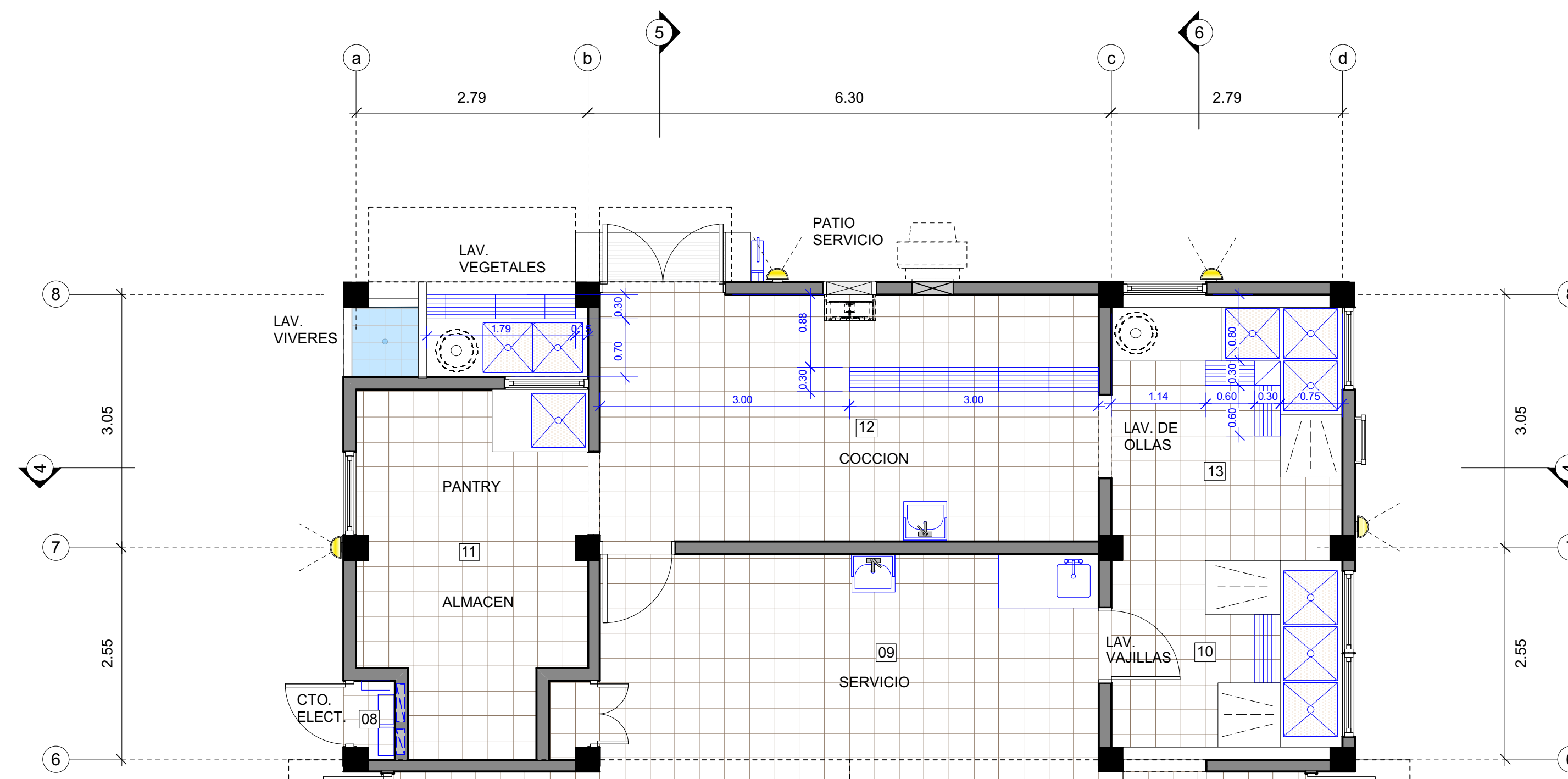
1 PLANTA DIMENSIONADA CANALETAS COCINA TIPO 1 Scale: 1:50
