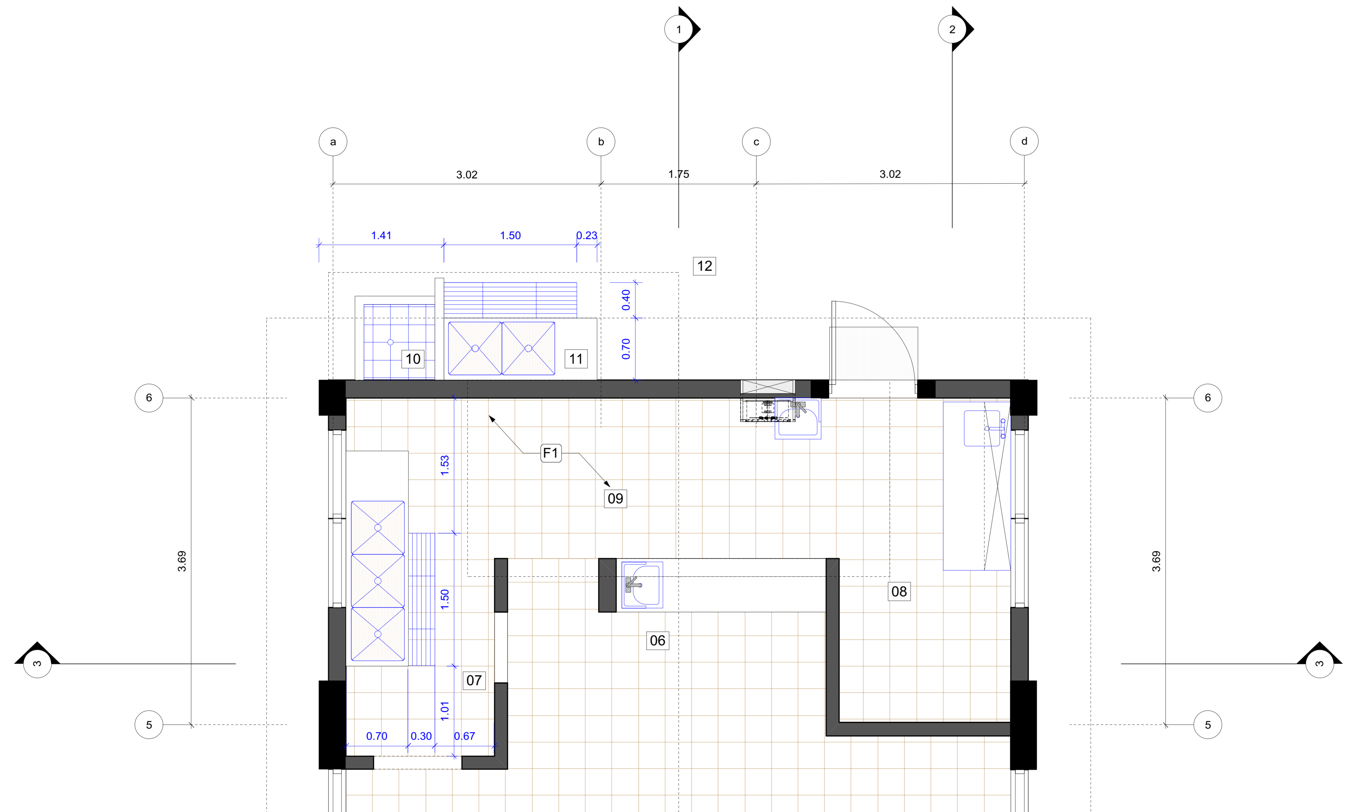
1 PLANTA DIMENSIONADA CANALETAS Scale: 1:25
