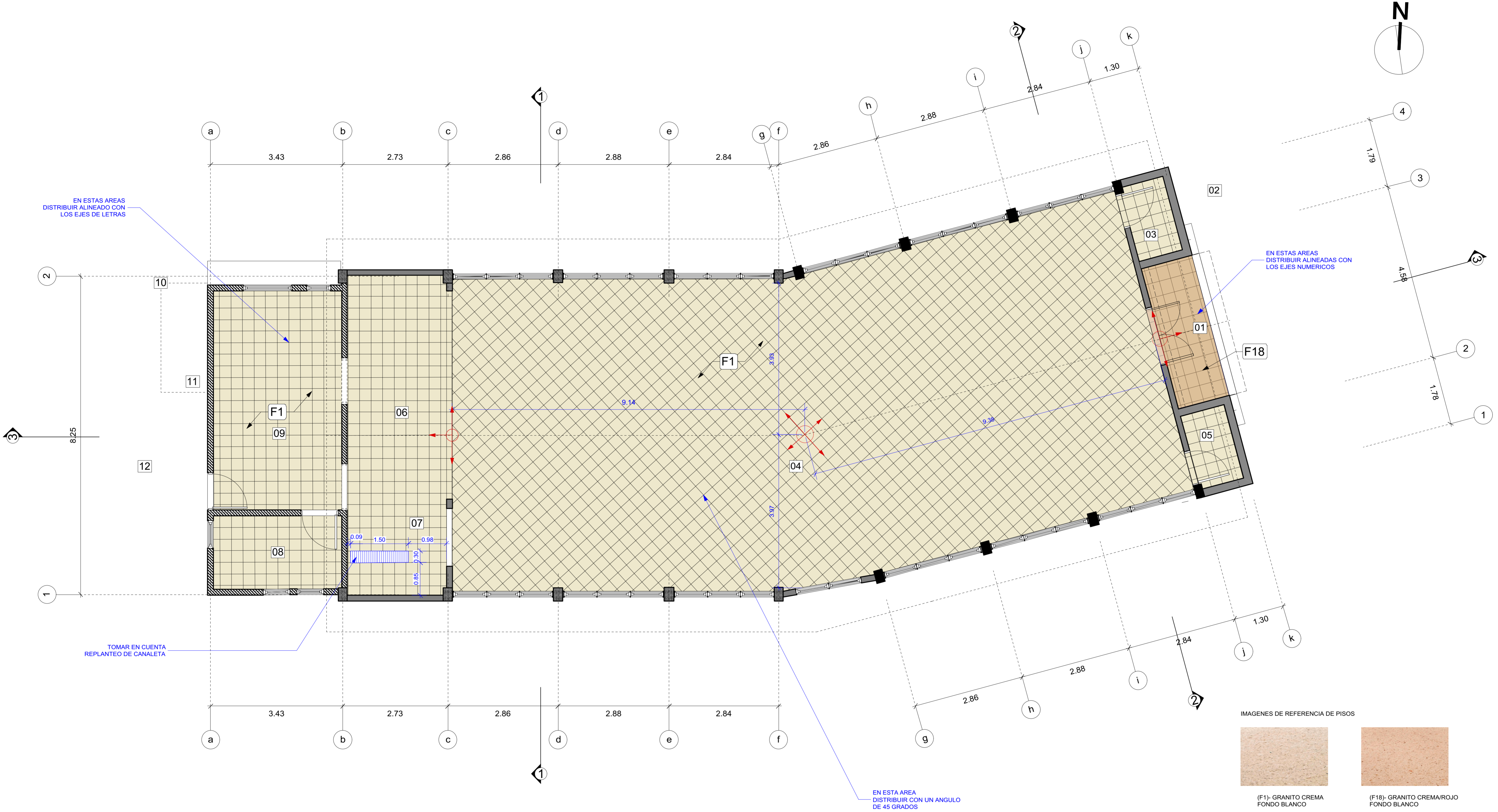
2 PLANTA ARQUITECTONICA AMUEBLADA Scale: 1:50
