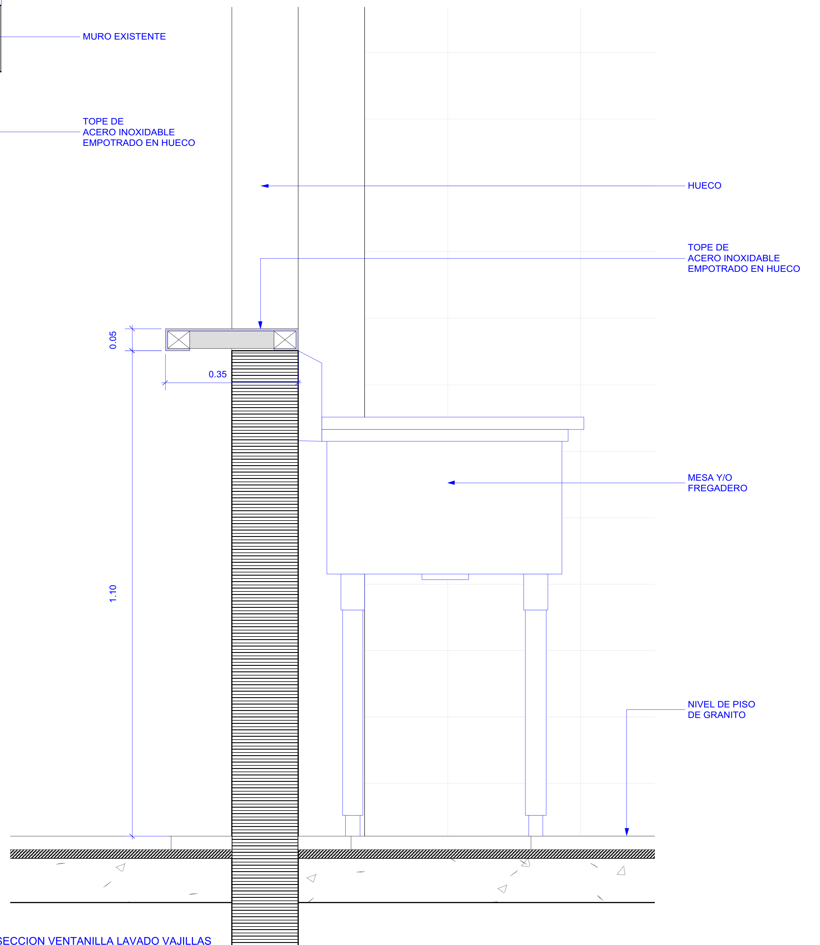
2 DETALLE TIPICO SECCION VENTANILLA LAVADO VAJILLAS Scale: 1:5
